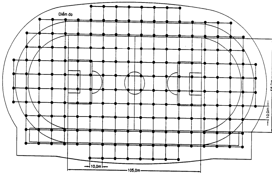
c. Hướng đo độ rọi đúng (Sân bóng đá)
