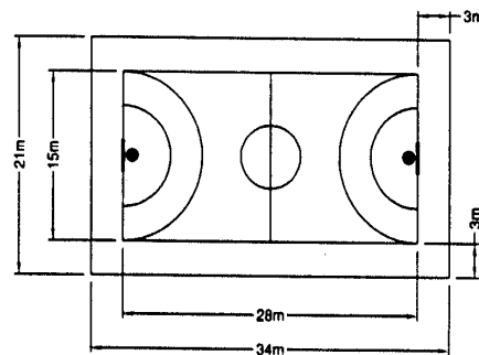
b. Sân bóng rổ
