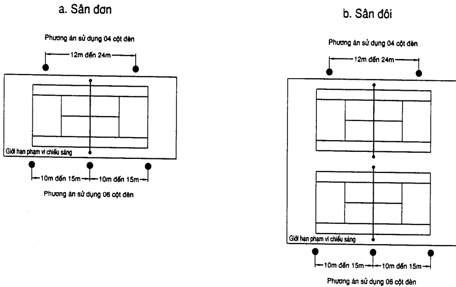
Hình 22 : Bố trí cột đèn chiếu sáng sân quần vợt không có hàng rào ngăn cách
