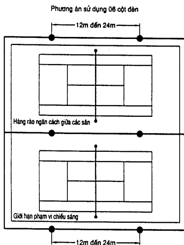
Hình 23 : Bố trí cột đèn chiếu sáng sân quần vợt có hàng rào ngăn cách
