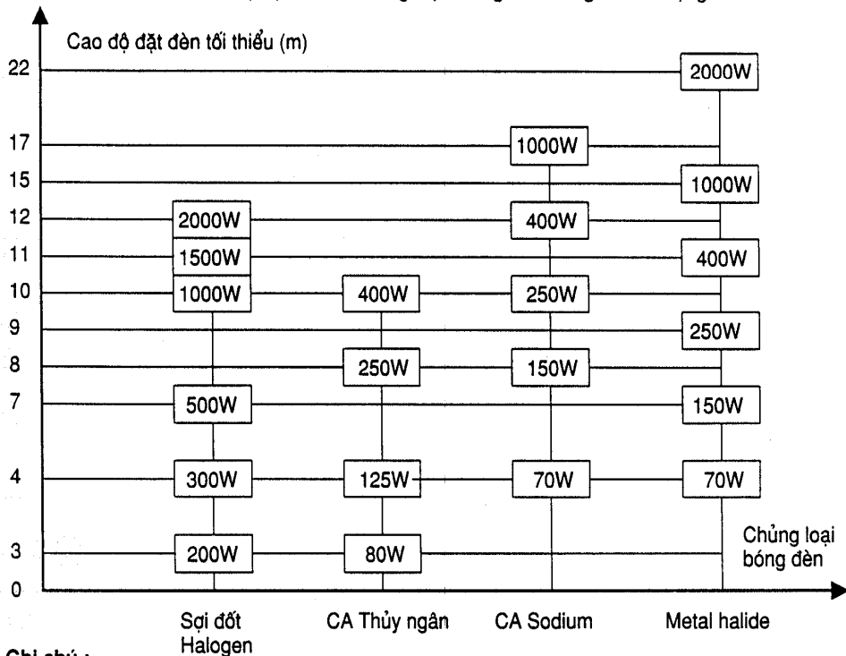
Hình 2 : Cao độ đặt đèn và chủng loại - công suất bóng đèn sử dụng
