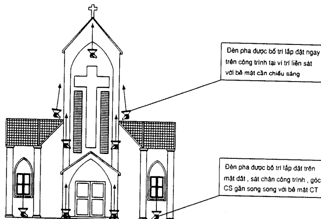
Hình 15 : Phương pháp bố trí chiếu sáng cục bộ
