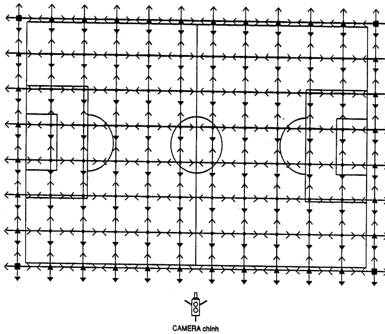
c. Hướng đo độ rọi đúng (Sân bóng đá)
