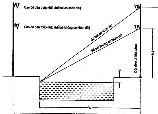
Hình 9 : Cao độ đặt đèn chiếu sáng bể bơi ngoài trời
