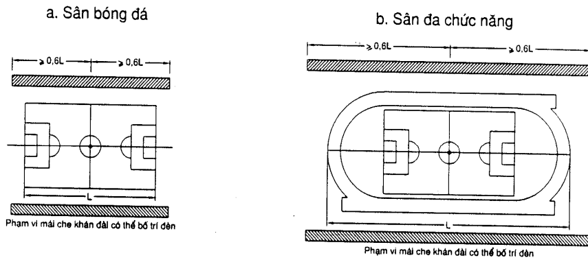
Hình 21 : Bố trí đèn chiếu sáng trên mái che khán đài
