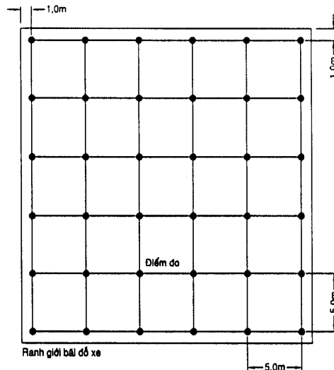
Hình 13 : Lưới đo kiểm chiếu sáng bãi đỗ xe ngoài trời
