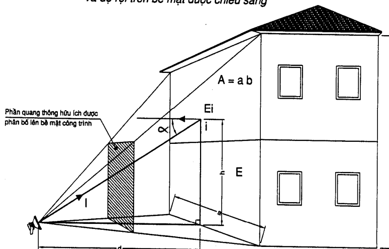
Hình 19 : Môi quan hệ giữa cường độ ánh sáng, khoảng cách chiếu sáng và độ rọi trên bề mặt được chiếu sáng
