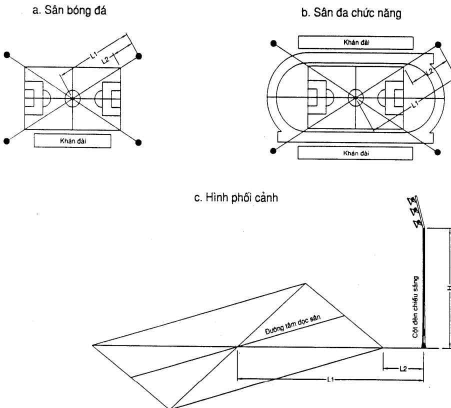
Hình 4 : Cao độ đặt đèn chiếu sáng sân vận động - trường hợp bố trí chiếu sáng bốn góc sân
