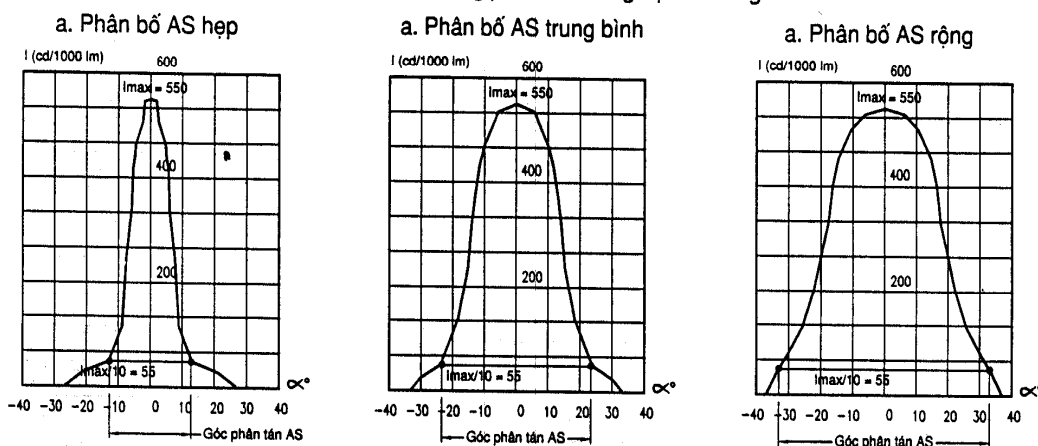
Hình 10 : Đường cong phân bố cường độ ánh sáng
