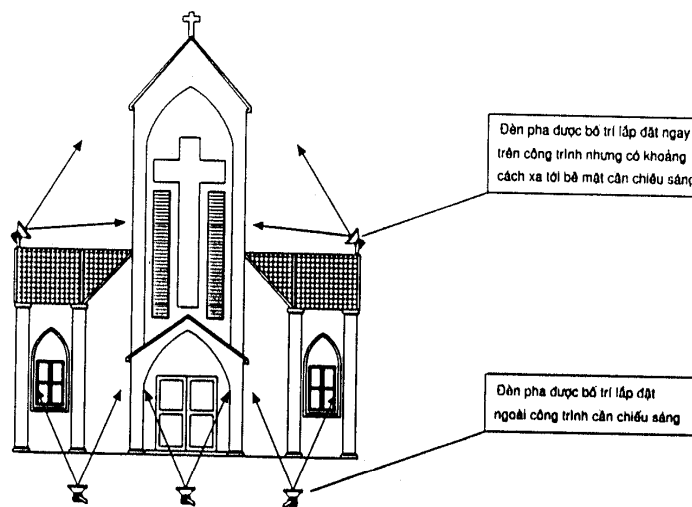
Hình 14 : Phương pháp bố trí chiếu sáng chung
