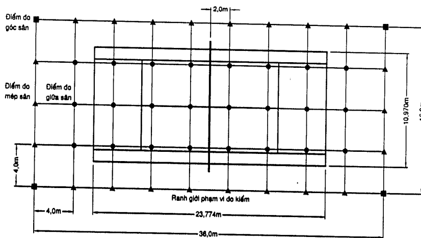
Hình 29 : Lưới đo kiểm chiếu sáng sân quần vợt
