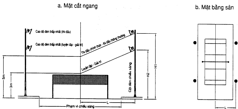
Hình 8 : Cao độ đặt đèn và khoảng cách chiếu sáng sân Bóng chuyền - Bóng rổ - Cầu lông
