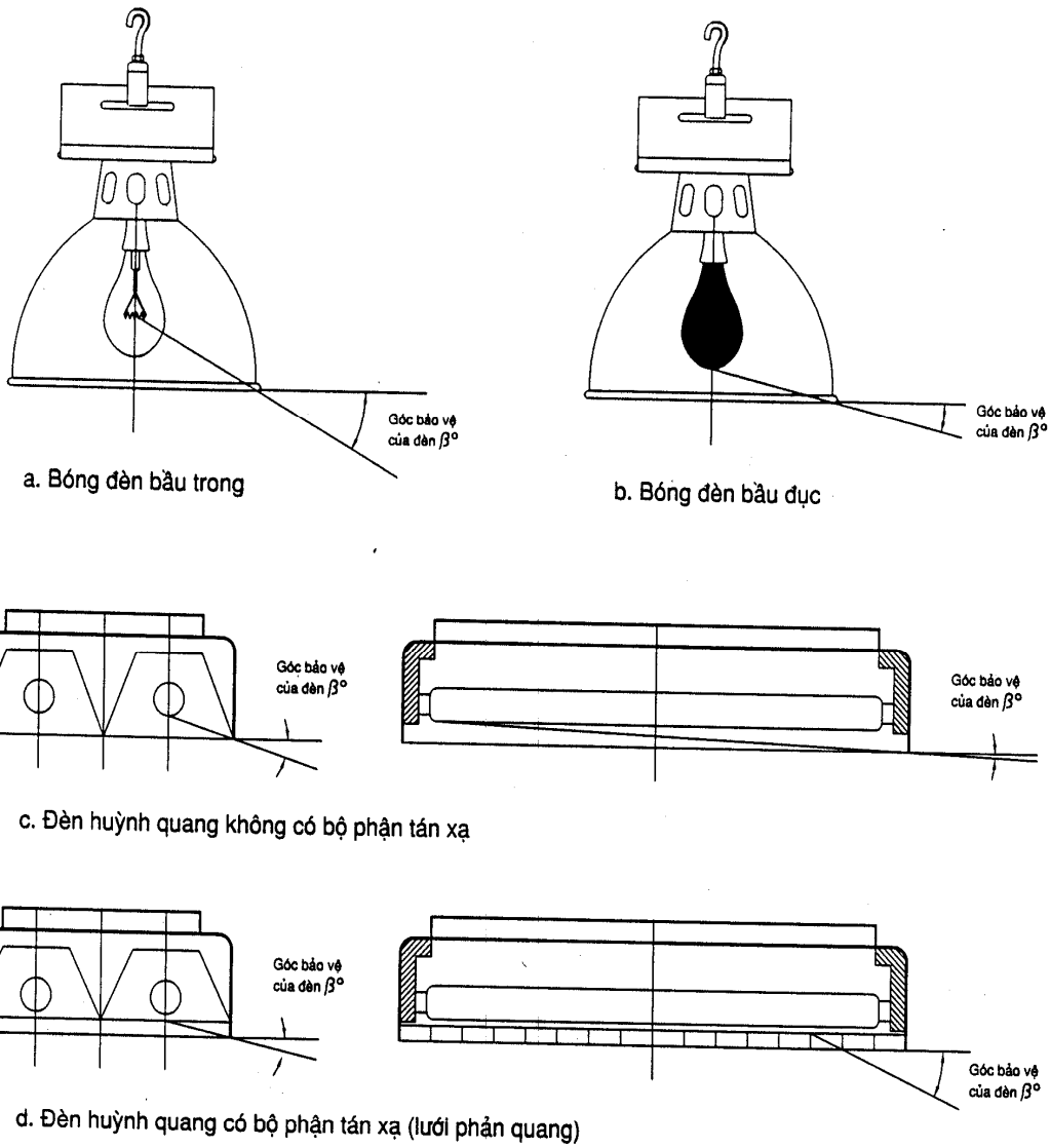
Hình 11 : Góc bảo vệ của đèn
